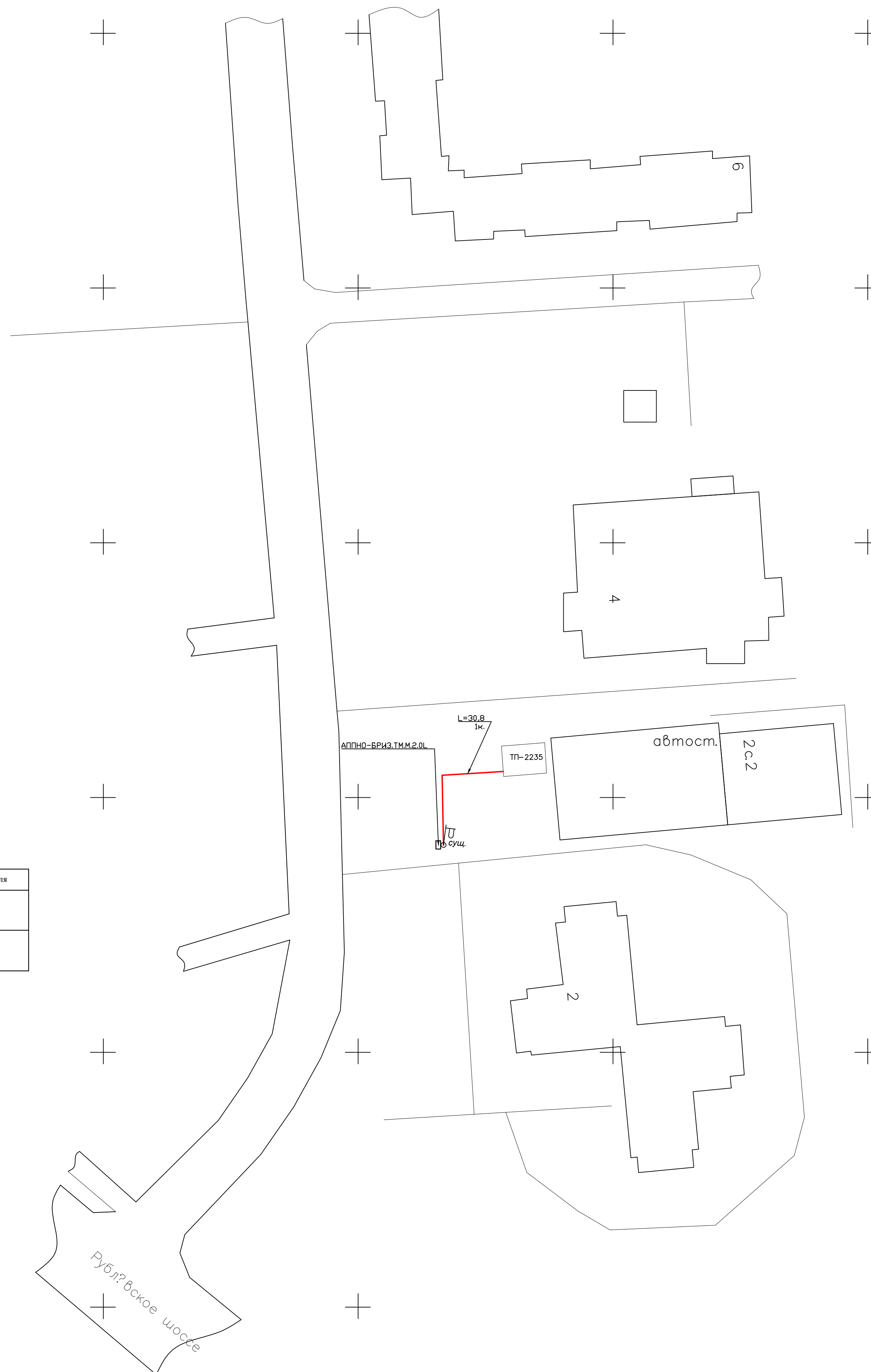
План наружного освещения М 1:500
